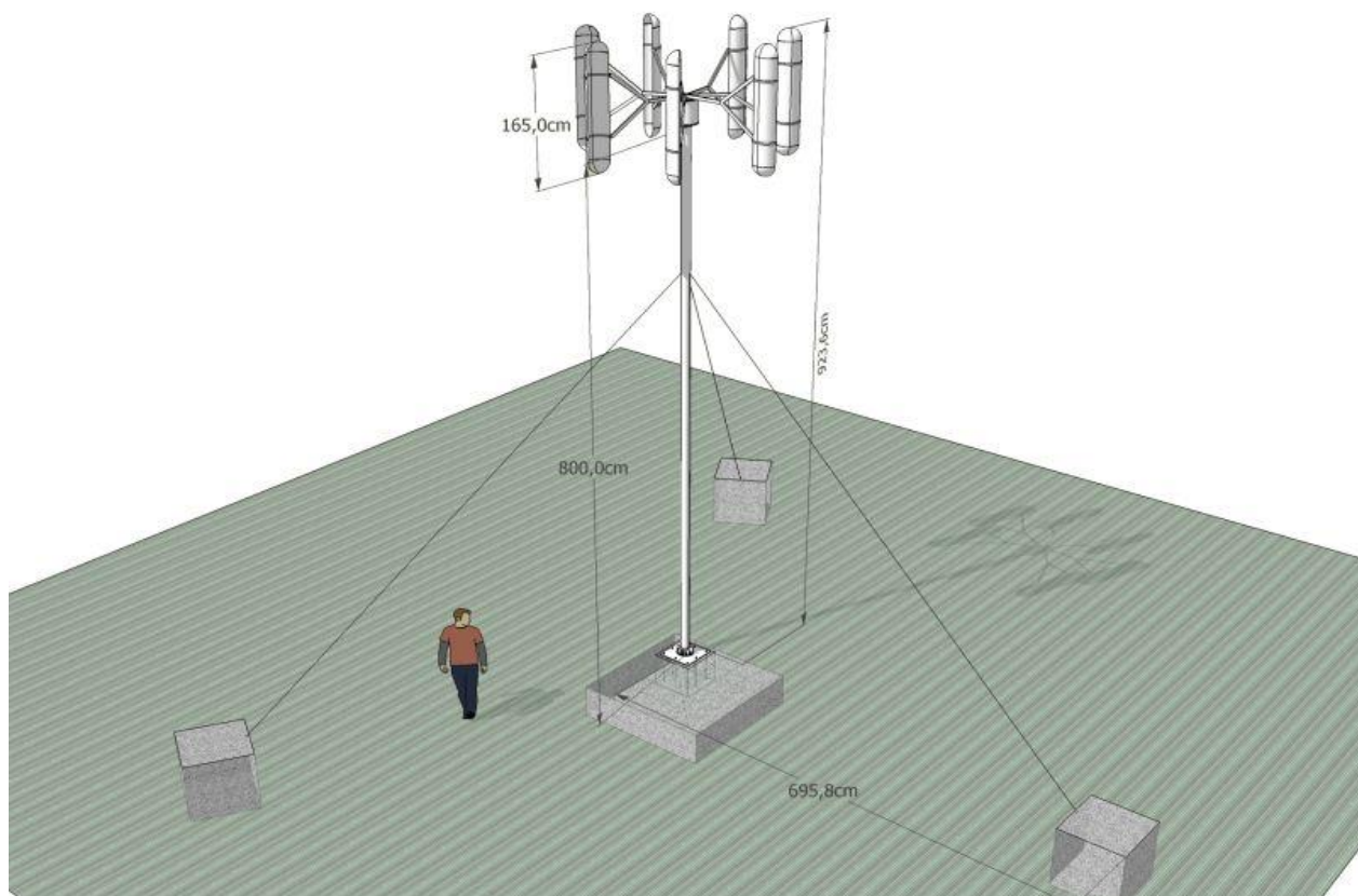
Rysunek 26. Parametry techniczne mikroturbiny wiatrowej ( http://generatory-wiatrowe.pl/?page_id=21 )
