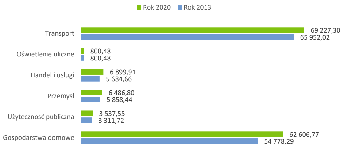
Rysunek 24. Graficzne zestawienie emisji CO 2 wg sektorów na terenie Gminy Szubin w roku 2013 oraz prognoza na rok 2020 (źródło: opracowanie własne)
